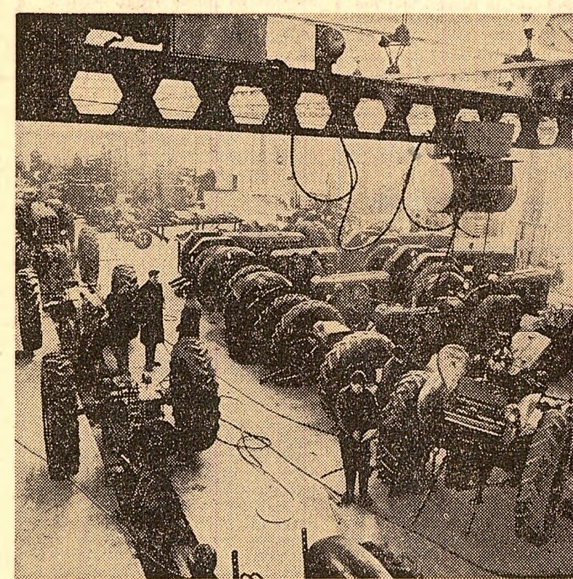
După cîteva săptămîni de la intrarea în funcțiune a primei linii tehnologice pentru tractoare și motoare a uzinei de reparatii din Bași (fotografia de mai sus) a început să producă cea de-a doua linie tehnologică. Proiectul de producție este organizat în flux continuu, automatizat, după tipul uzinei de tractoare din Brașov. Noua întreprindere din Bași va putea repara anual 3.400 de motoare și 1.200 de tractoare, concomitent cu producerea și recondiționarea a circa 800 tone de piese de schimb și 1.000 tone de utilaje necesare diferitelor tipuri de mașini agricole. Uzina este considerată a fi una dintre cele mai moderne de acest fel din țară.
