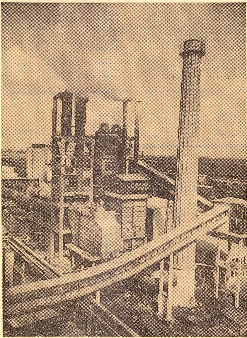
În cadrul lucrărilor de extindere a capacităților uzinei de aluminiu din Oradea s-a construit un nou cuplor de caldănat cu o producție de 17 tone pe oră
