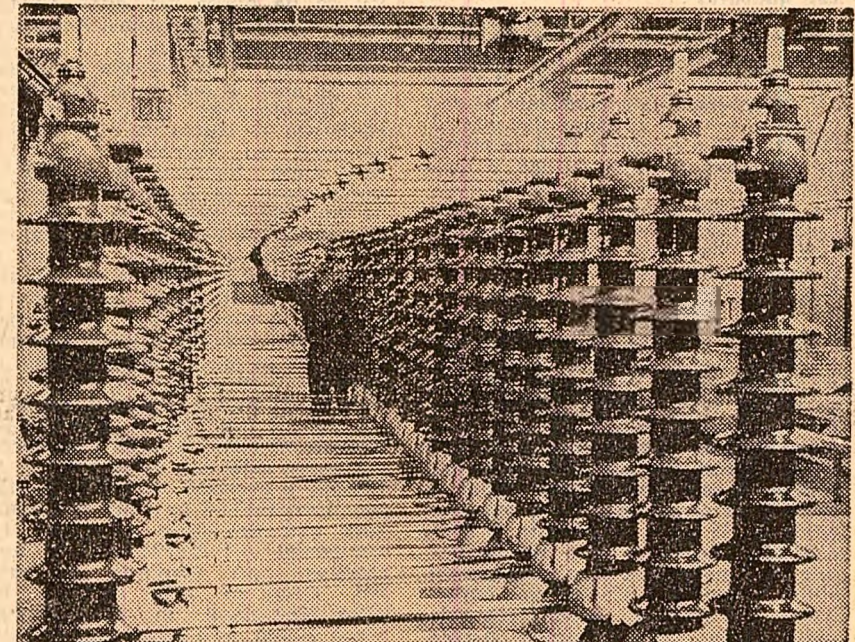
Uzina „Electropulere” Craiova. Aspect din atelierul separatori de exterior utilizați în rețelele electrice
