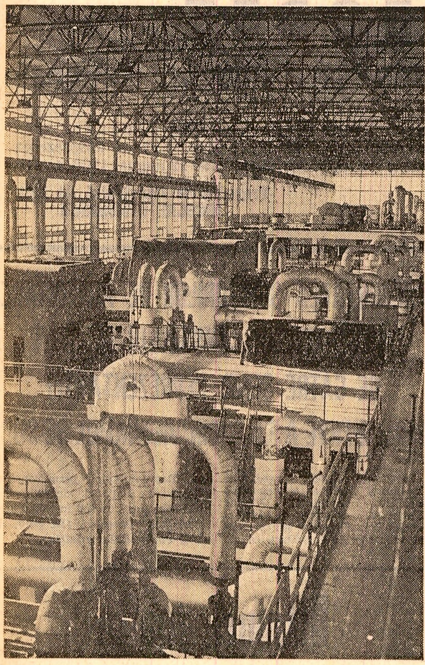
Hala turbinelor de la termocentrala Işalniţa
