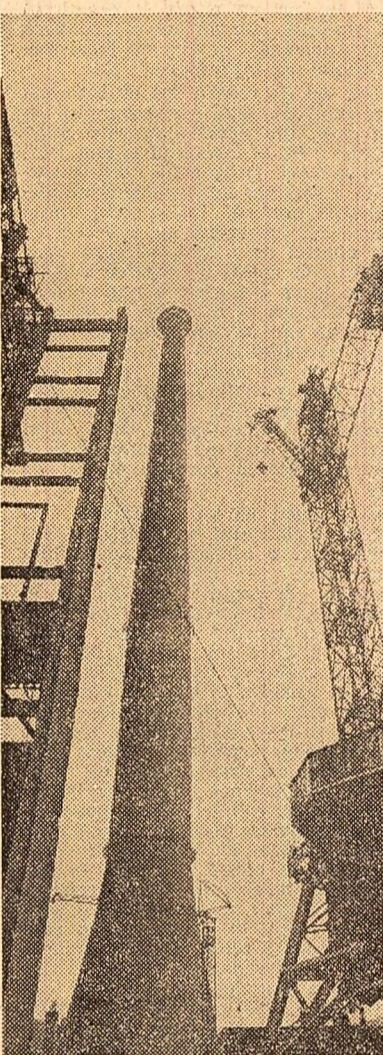
Coșul de fum al centralei electrice de termoficare a la Deva. Constructorii au încheiat cu 12 zile mai devreme, față de grafic, gisarea celei mai înalte construcții din țară — 220 metri. A fost întrecut, astfel, cu 20 de metri, recordul de înălțime deținut pînă acum de construcția agmînditoare de la Craiova
