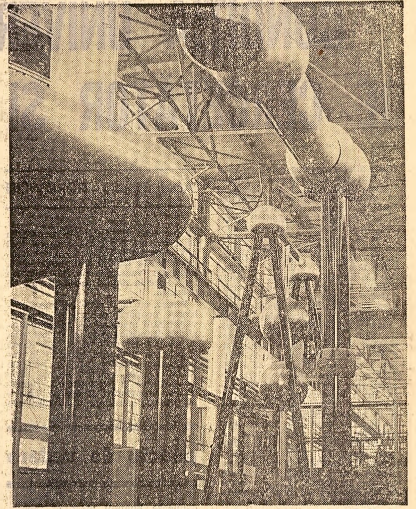
Standul de probă al aparatelor de înaltă tensiune de la uzina „Electroputere” Craiova (Foto: Gh. Vințilă)
