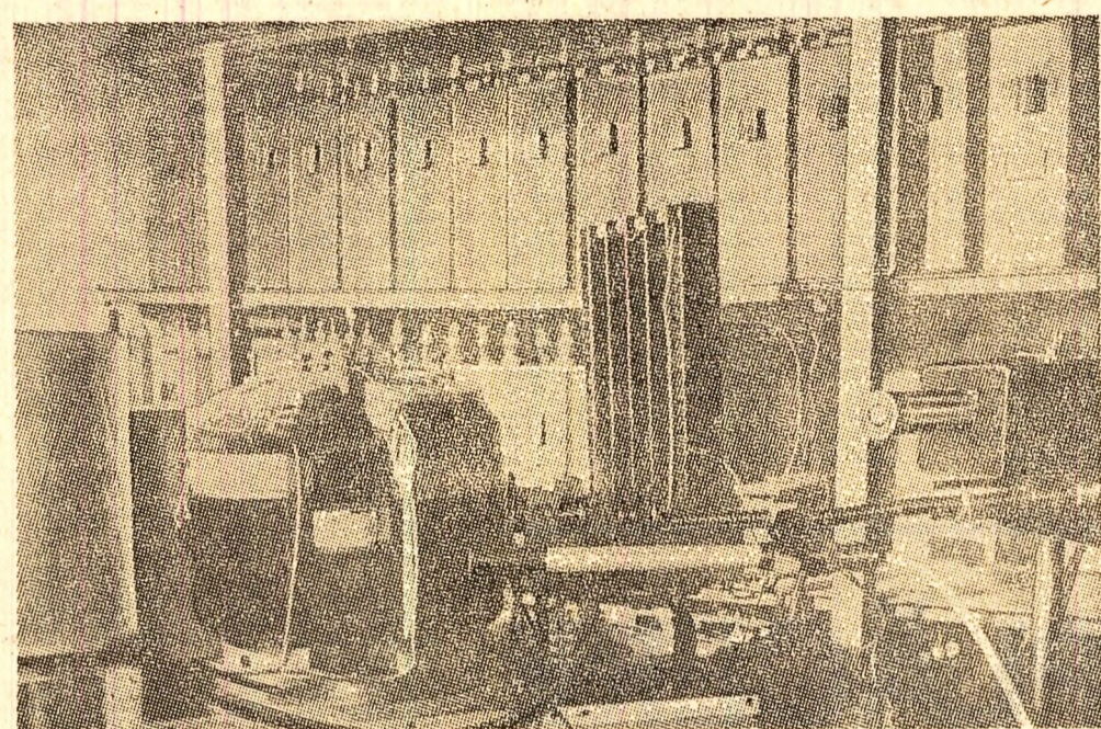
Beatronul de 8 MeV al Institutului de Fizică Atomică, al doilea accelerador de particule de acest tip conceput și realizat în întregime de specialiști români, este utilizat pentru cercetări de fizică și pentru controlul nedestructiv al unor piese sudate sau turnate
