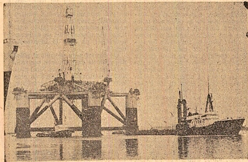
„Petrol 81” este cea mai mare platformă construită în Franța pentru cercetări petroliere sub marine. În fotografie: platforma este transportată din portul Le Havre spre golful Gasconia
