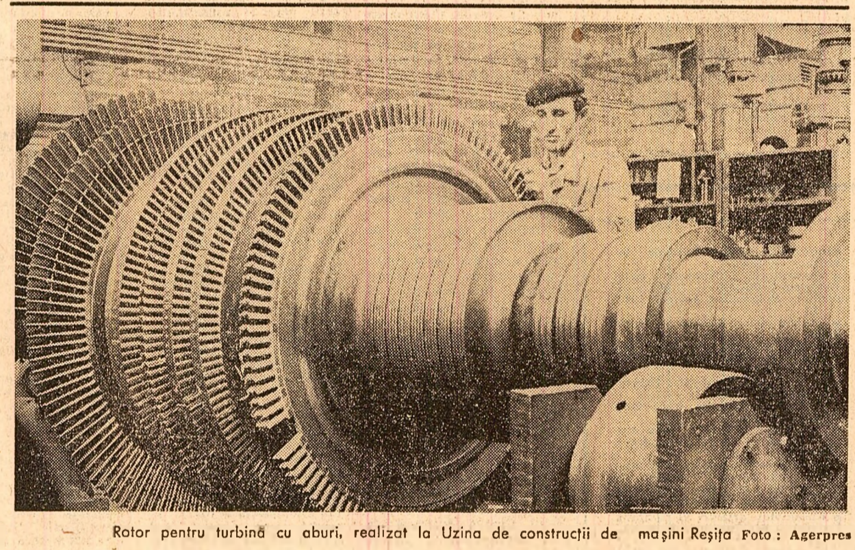
Rotor pentru turbină cu aburi, realizat la Uzina de construcţii de maşini Reşiţa. Foto: Agerpres
