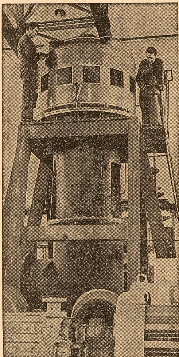
D.V.R. 5-110 — un nou tip de pompă de mare capacitate — va intra în curând în fabricație de serie la Uzina de pompe din București. Proiectată pentru instalații de hidroamploraj, pompa are un debit de 14 000 la 23 000 m.c. de apă pe oră
