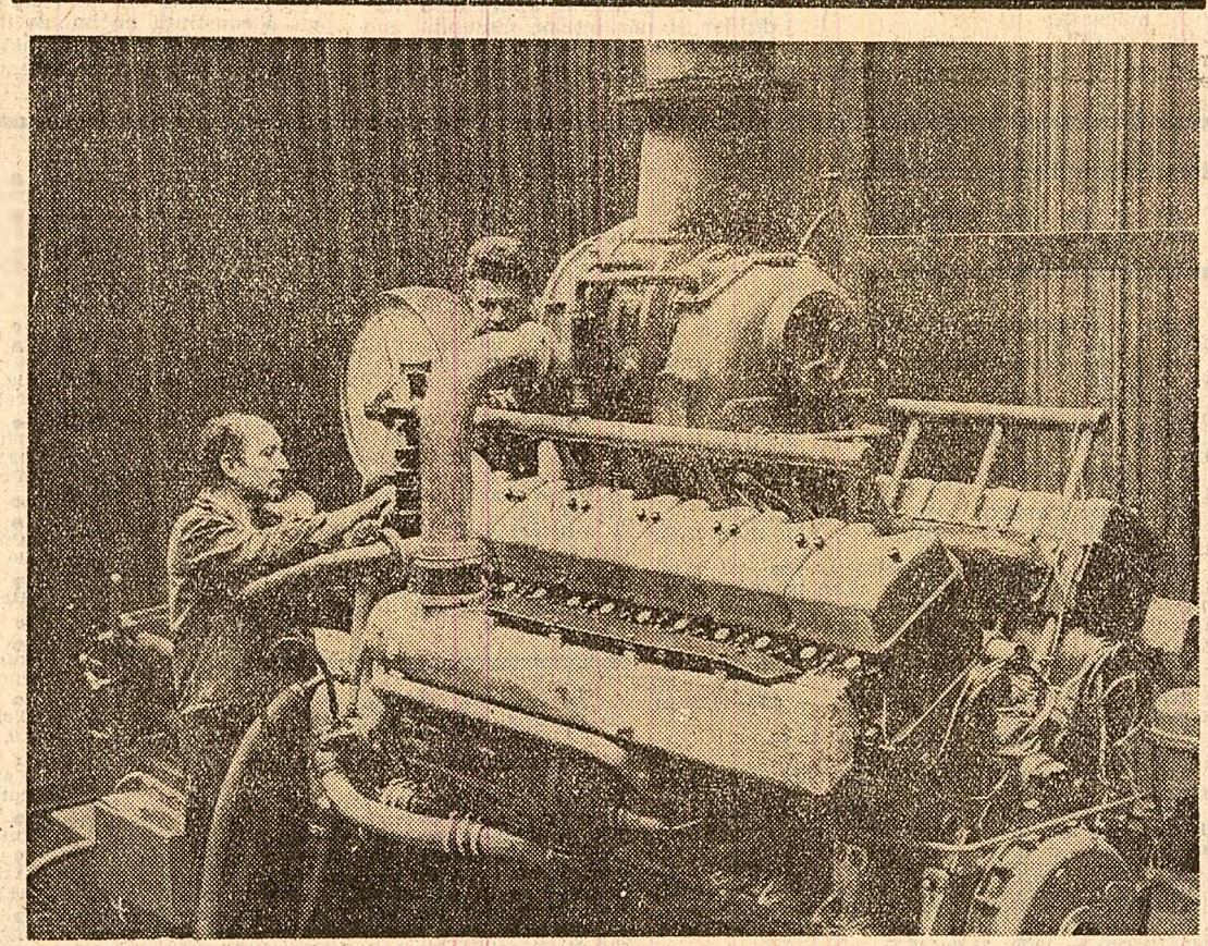
Uzinele „23 August” din Capitală: Motorul de 700 CP. M-12 la bancul de probe
