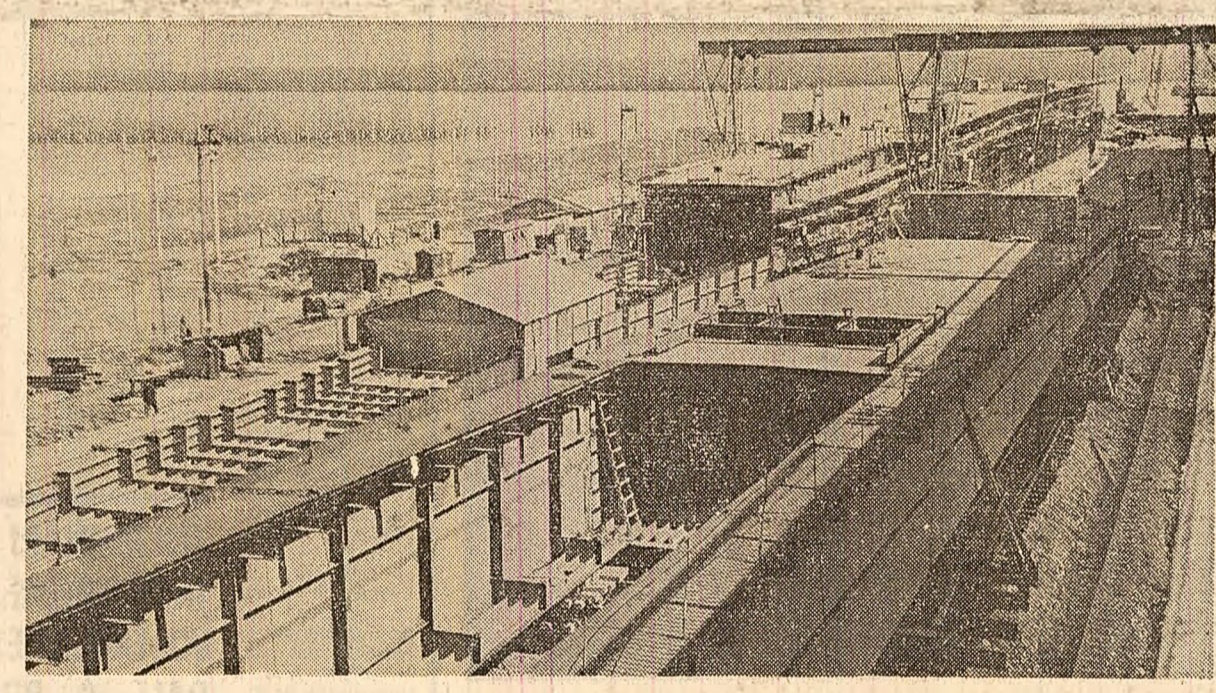
Pe șantiul celui mai mare pod rutier din țara noastră, Giurgeni—Vadul Oii, se înregistrează cu fiecare zi contururi tot mai precise. Foto: Agerpres
