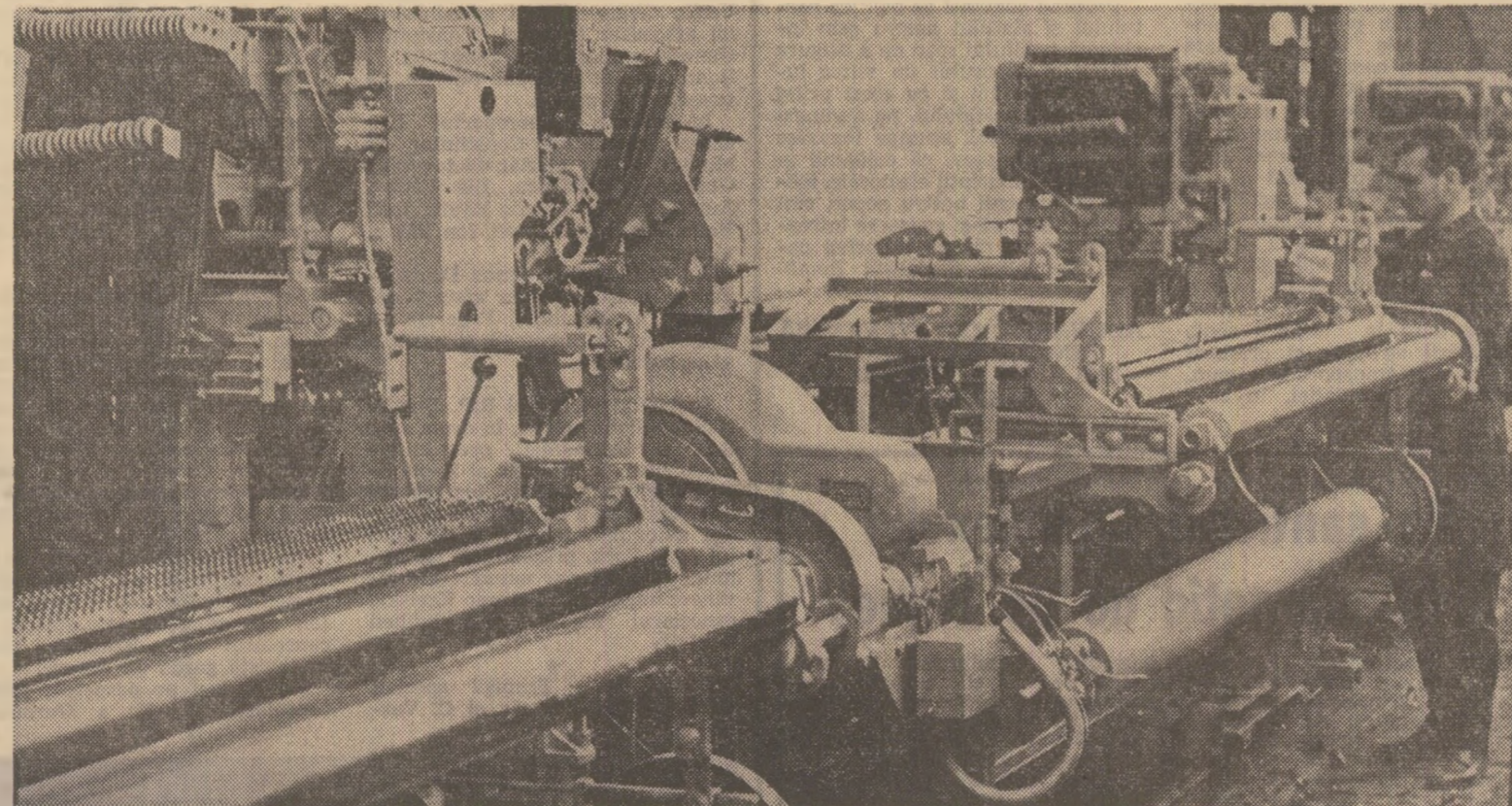
La întreprinderea de utilaje pentru industria ușoară din Tîrgu-Mureș recuperarea timpului furat de ape se conjoagă cu eforturile consacrate îndeplinirii angajamentelor suplimentare. Noi mașini textile părăsesc montajul
