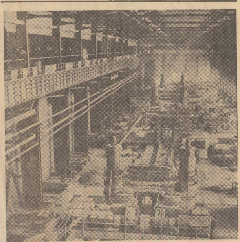
La Combinatul siderurgic Galați se află în plină construcție laminorul de benzi la cald. În fotografie: hala noului laminor — zona cailor Foto: M. Andreescu
