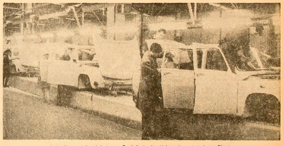
Linia de montaj auto-lurisme „Dacia” de la Uzina de autoturisme Ploiești
