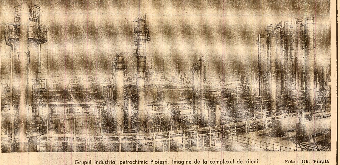
Grupul industrial petrochimic Ploiești. Imagine de la complexul de xileni Foto: Gh. Vîniță
