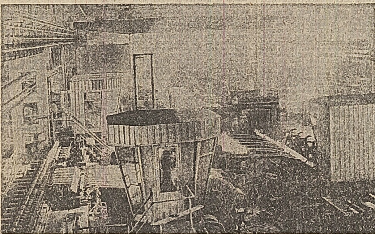
Laminorul de 4 jolii al Uzinei de țevi din Roman.
