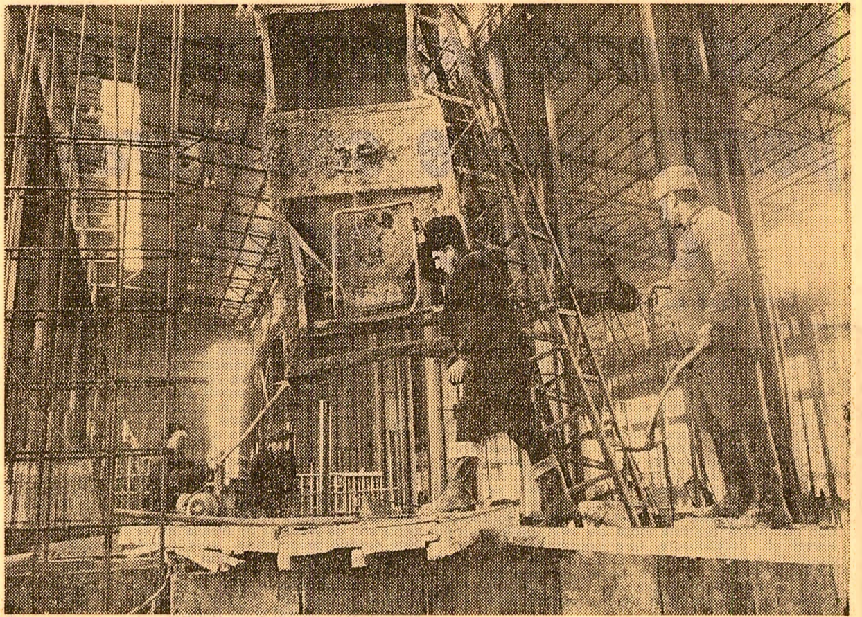
Constructorii oţelăriei electrice nr. 2 de pe platforma industrială Tîrgovişte s-au angajat să devanseze termenul final de punere în funcţiune a primului cuplor de 50 tone, din trimestrul IV în trimestrul III a.c. în fotografie: echipa de betonişti condusă de Ion Văduvoiu, lucrînd la turnarea betonului pentru cuplorul nr. 3. Foto: S. Cristian
