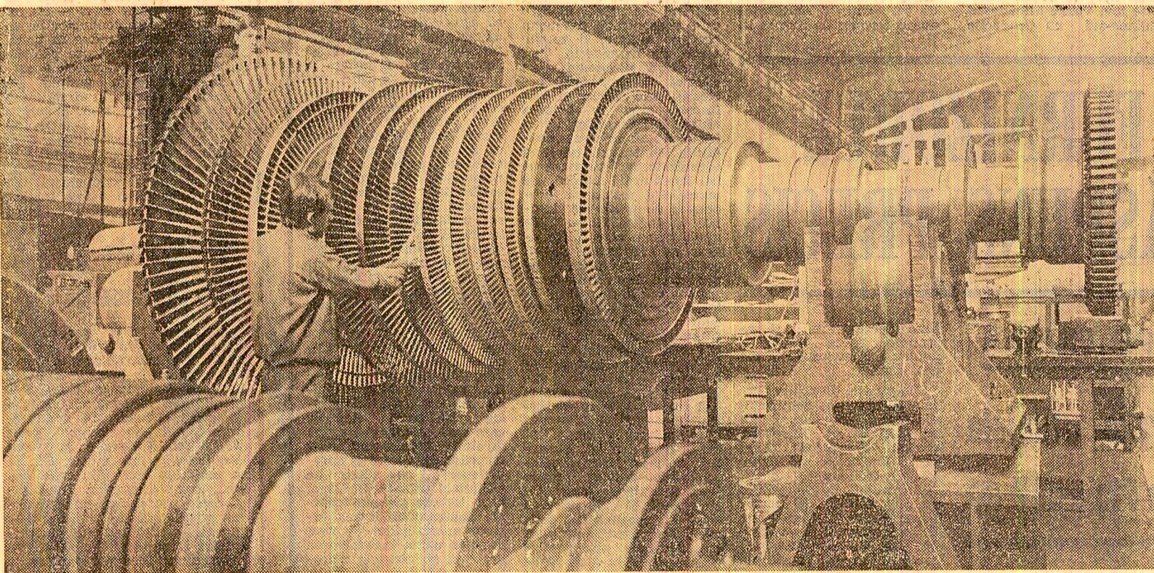
Nu peste mult timp, în imediata apropiere a platformei chimice de la Rm. Vilcea, la centrala termoelectrică de la Govora, se va monta această piesă de mari proporţii, dar şi de mare fineţe şi precizie: rotorul unei turbine de 50 MW. Piesa aceasta de maximă importanţă, aflată deocamdată — după cum se vede în fotografie — în curs de execuţie la Uzina constructoare de maşini din Reşiţa, constituie încă unul din motivele de mîndrie ale colectivului acestei mari uzine, care nu o dată a izbucnit performanţelor unor agregate de mari dimensiuni şi de uimitoare precizie necesare noilor obiective hidro şi termoelectrice construite în ţara noastră. Foto: E. Dichişeanu
