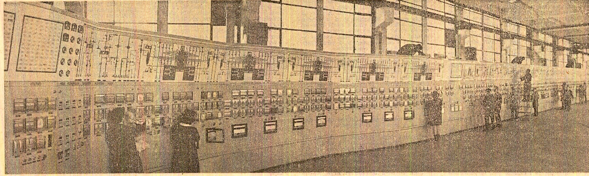
La întreprinderea „Automatică” din București se execută ultimele controale tehnice la instalația de automatizare pentru „Piraliză II” — destinată grupului industrial de petrochimie Pitești
