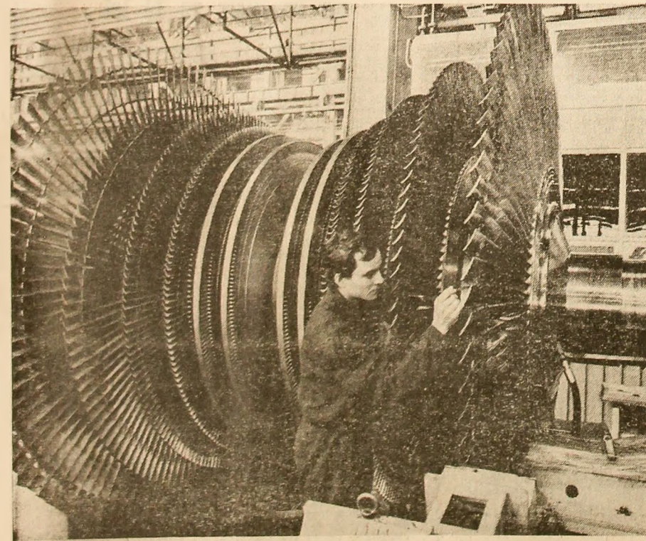
Imagine din moderna Uzină de mașini grele din București
