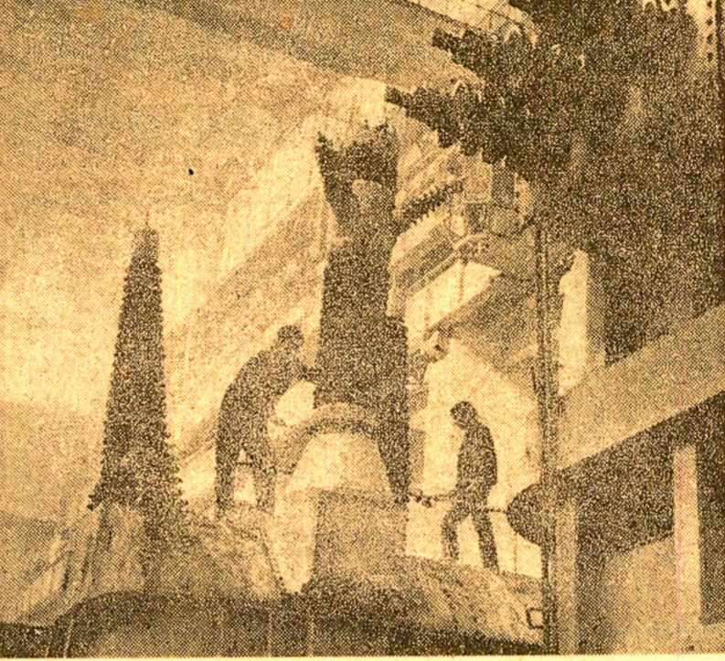
La uzina „Electropulere” din Craiova se realizează în acest an aproape 40 de transformatoare de puteri mari. În fotografie: se lucrează la transformatorul de 200 MVA destinat platformei industriale de la Tîrgoviște
