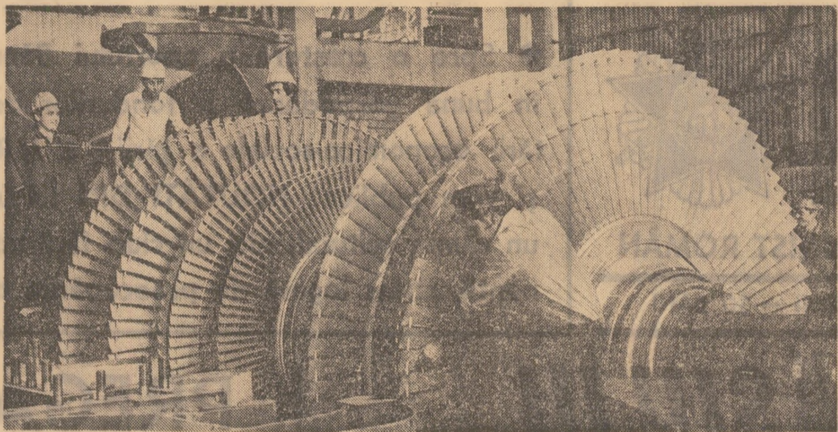
La termocentrala Brăila se montează una dintre turbine. Foto: N. Moldoveanu
