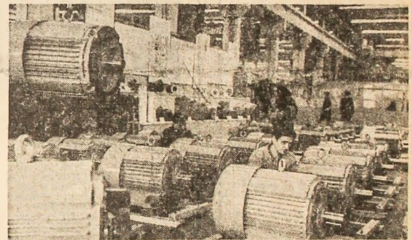
ÎNTEPRINDEREA DE MAȘINI ELECTRICE. Harnicul colectiv de muncitori al unității bucureștene a îndeplinit planul pe primii trei ani ai cincinalului cu 90 de zile înainte de termen. În fotografie: un aspect al finisării motoarelor A.S.I. 280
