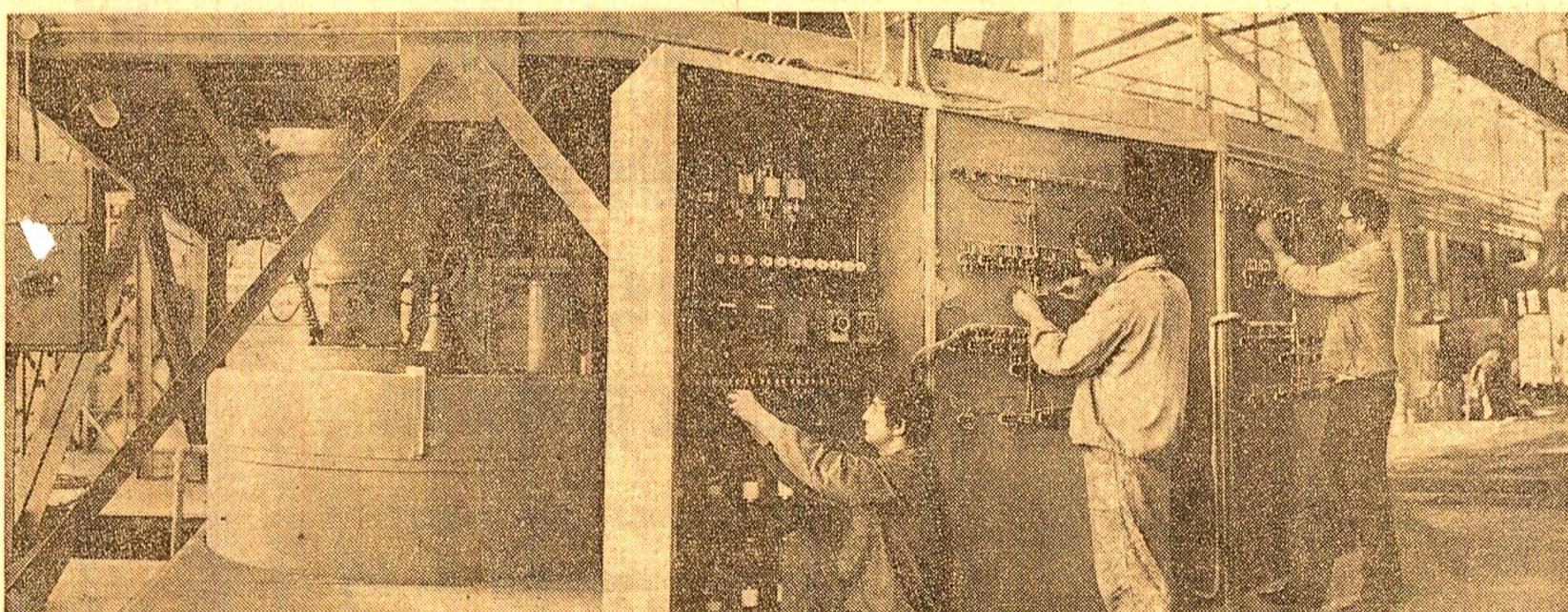
Pentru grăbirea punerii în funcțiune a turbinelor de fontă de la Vulcan—București, constructorii de la ICSIM—București fac ultimele verificări la tabloul de comandă al ansamblului mecanizat. Foto: S. Cristian
