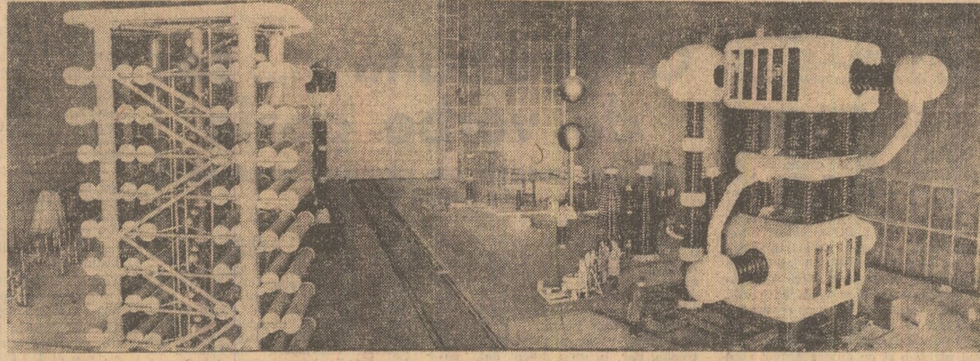
Întreprinderea „Electroputere” Craiova: laboratorul de înaltă tensiune. Foto: E. Dichiseanu
