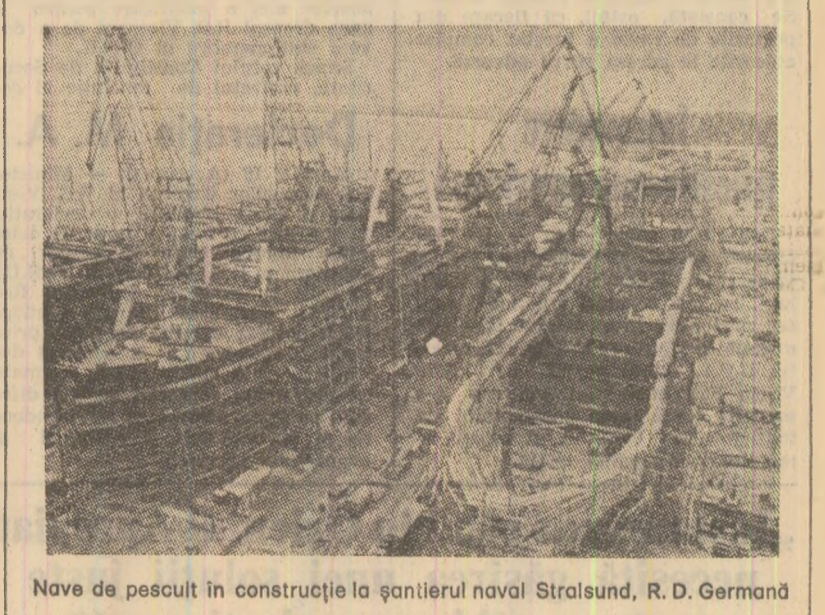
Nave de pescuit în construcție la șantierul naval Stralsund, R. D. Germană
