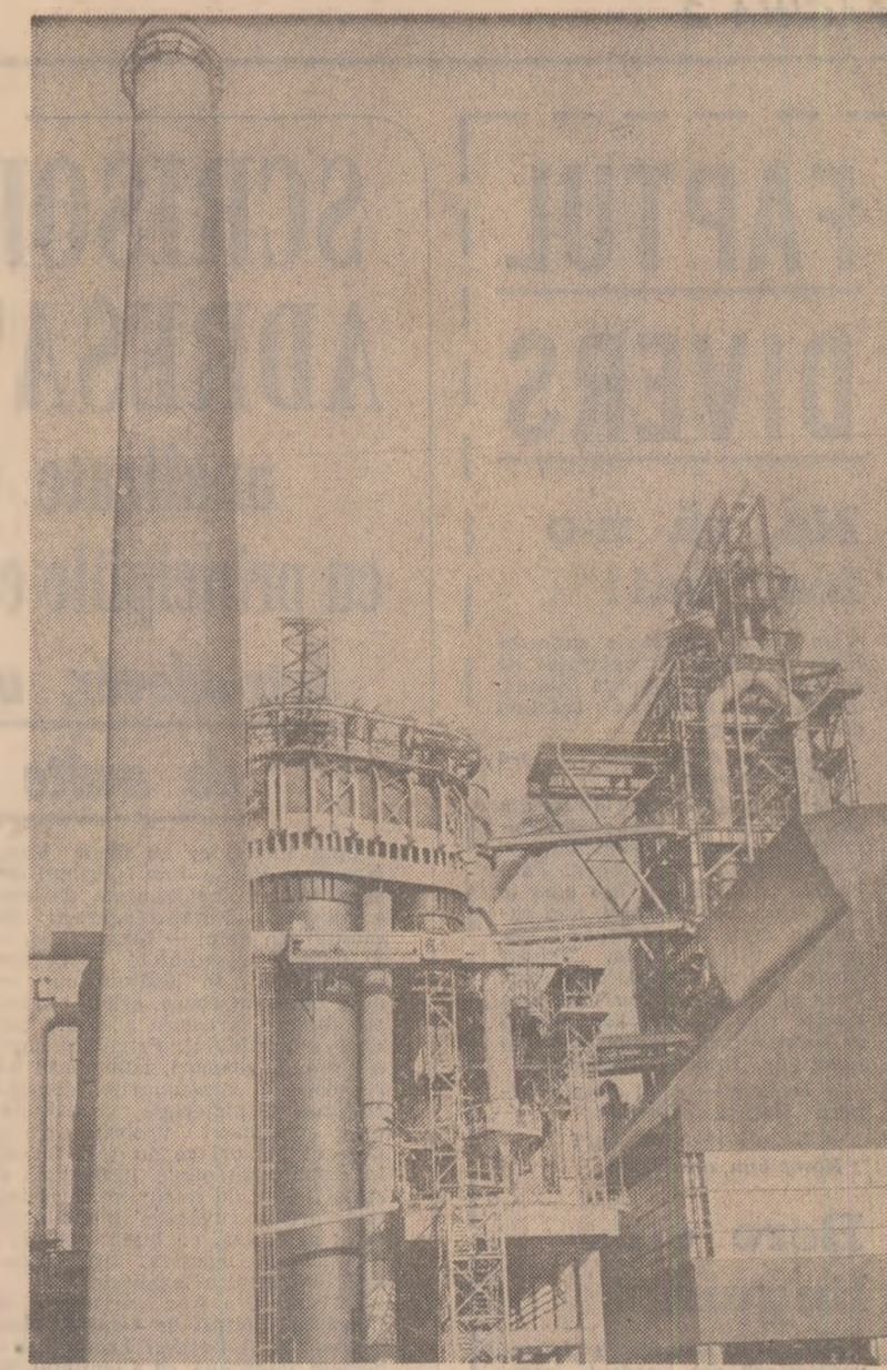
Furnalul nr. 5, de 2700 mc (din fotografie), de la Combinatul siderurgic — Galați deține, pînă la ora actuală, recordul de putere între furnalele României. Pînă la ora actuală, deoarece îl va deținea, încă în acest an, furnalul nr. 6, de 3500 mc. Reportajul de față este consacrat vieții și muncii de fiecare zi a constructorilor acestui mare obiectiv al cincinalului.
