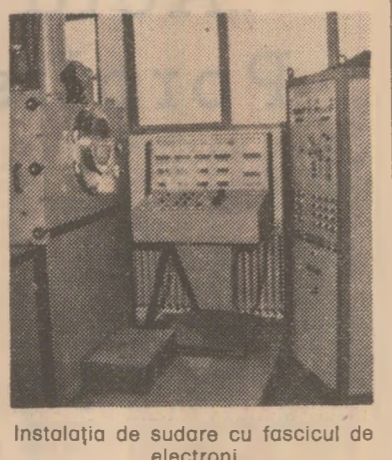
Instalația de sudare cu fascicul de electroni
