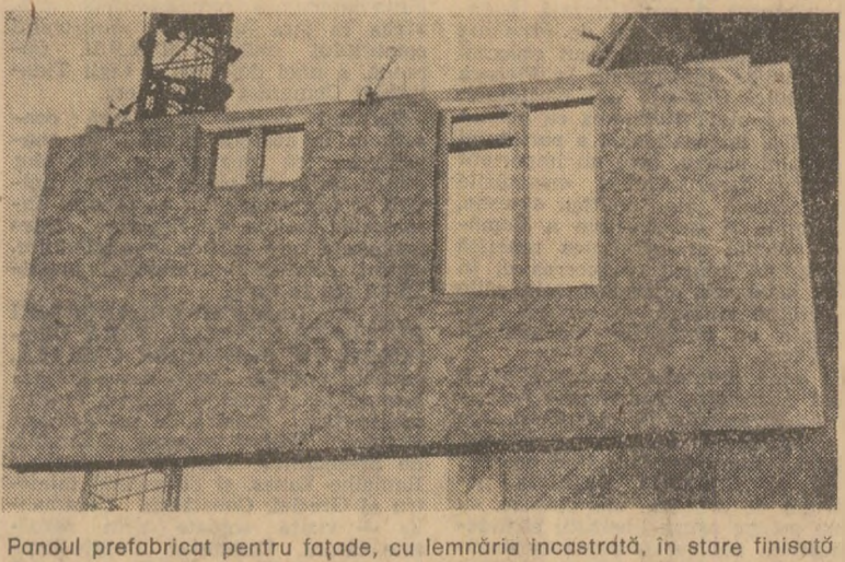
Panoul prefabricat pentru fațade, cu lemnăria încastrată, în stare finisată
