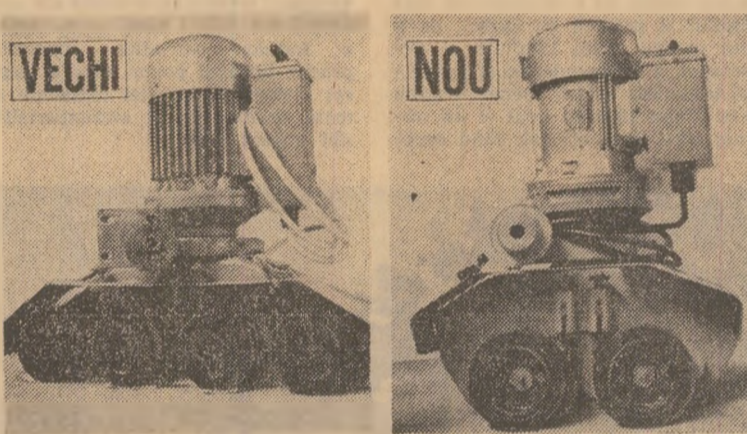
În unitățile Centralei de Utlaje și piese de schimb București se preconizează ca, prin reproiectări și modernizări, tehnologii moderne, utilizarea de materiale noi ș.a., să se obțină în 1980 o economie, față de normele inițiale, de peste 33 000 tone metal. Iată unul din aceste utlaje — dispozitivul de avans mecanic — înainte și după reproiectare; în varianta nouă, consumul de metal este cu 40 la sută mai redus.
