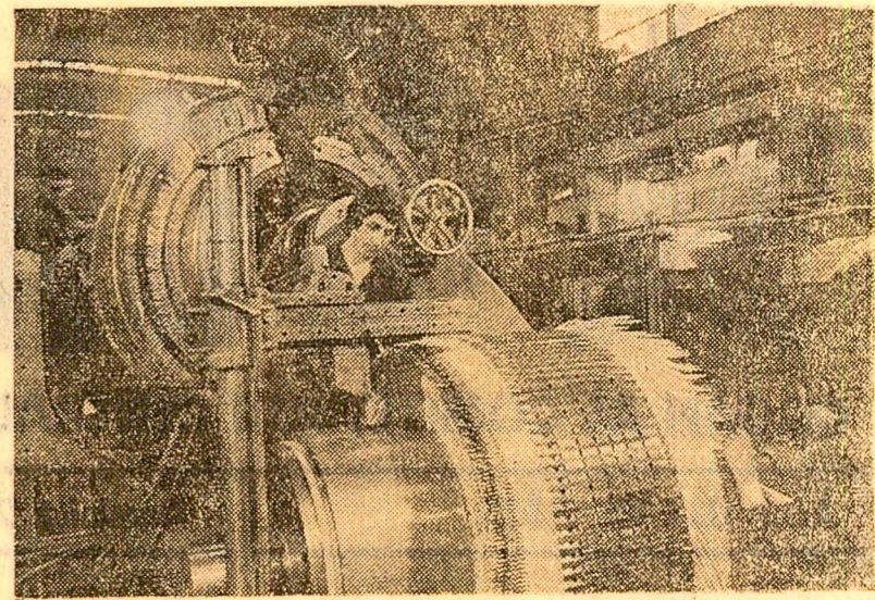
La întreprinderea de construcții de mașini din Reșița a fost asamblat în producție un nou motor electric de curent continuu de 2.500 kW
