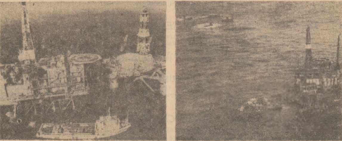
În zona norvegică a zăcămintului petrolifer Ekofisk din Marea Nordului a fost răsturnată de furtună platforma „Alexander Kielland” (în partea stângă — fotografie realizată înainte de catastrofa). În imaginea din dreapta se văd cele patru stilpi pontoni ai platformei după răsturnare
