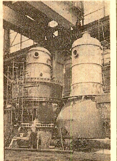
Doi tronsoane ale coloanei pentru instalatiile de distilare a fițeiului in vid, oprite pe stindul de montaj al secției cozonerie de la întreprinderea de utilaj chimic „Grivița roșie” — București
