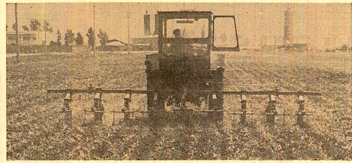
Întreținerea mecanică a culturii de porumb (însămînțată după recoltarea orzului), la I.A.S. Redea, județul Olt. Foto: E. Dichisneanu
