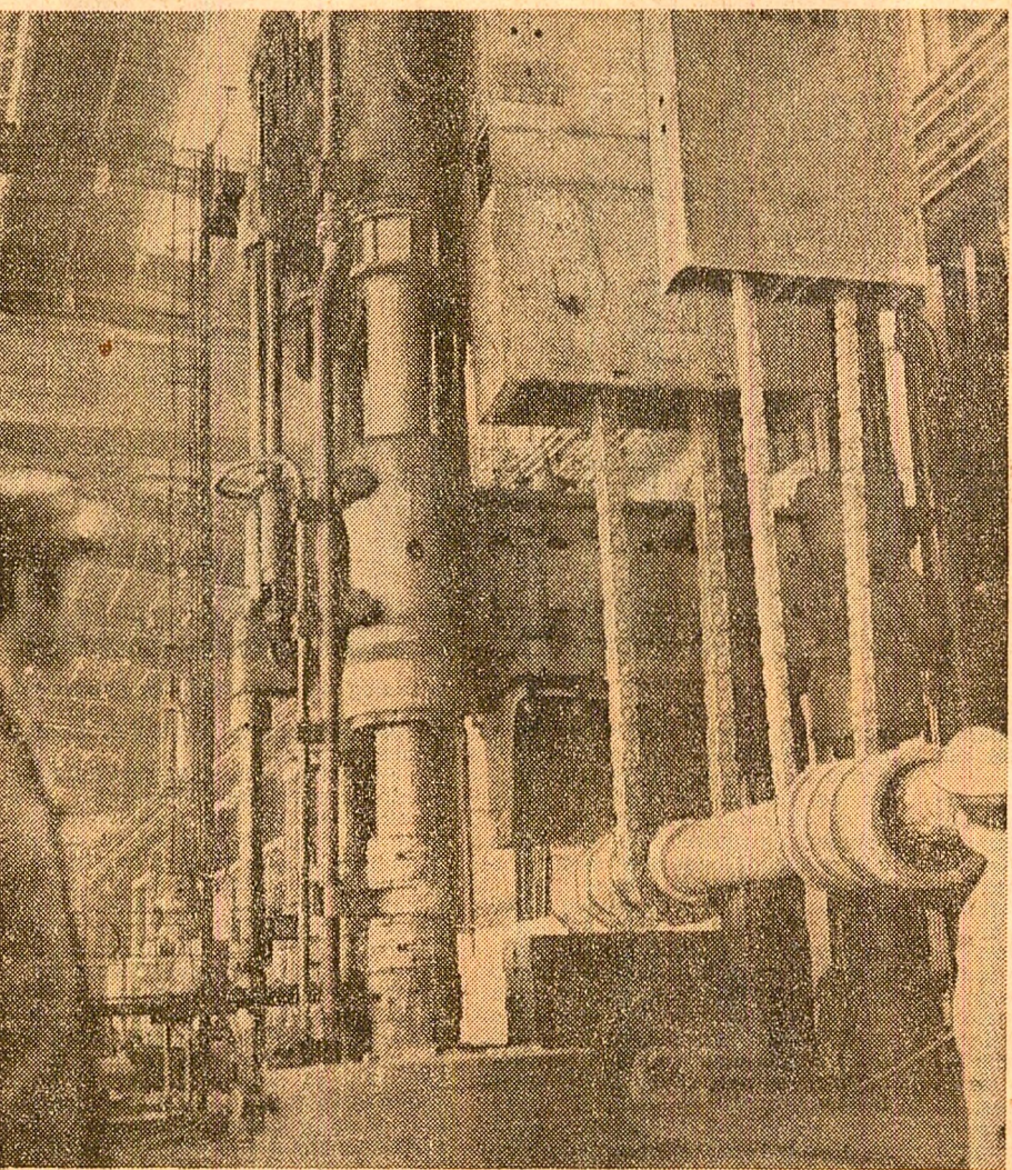
Multe sint utilajele unicate la această prestigioasă unitate industrială. Intre ele, un loc aparte îl ocupă presa de 12 000 tone/forță, creație a inteligenței tehnice românești
