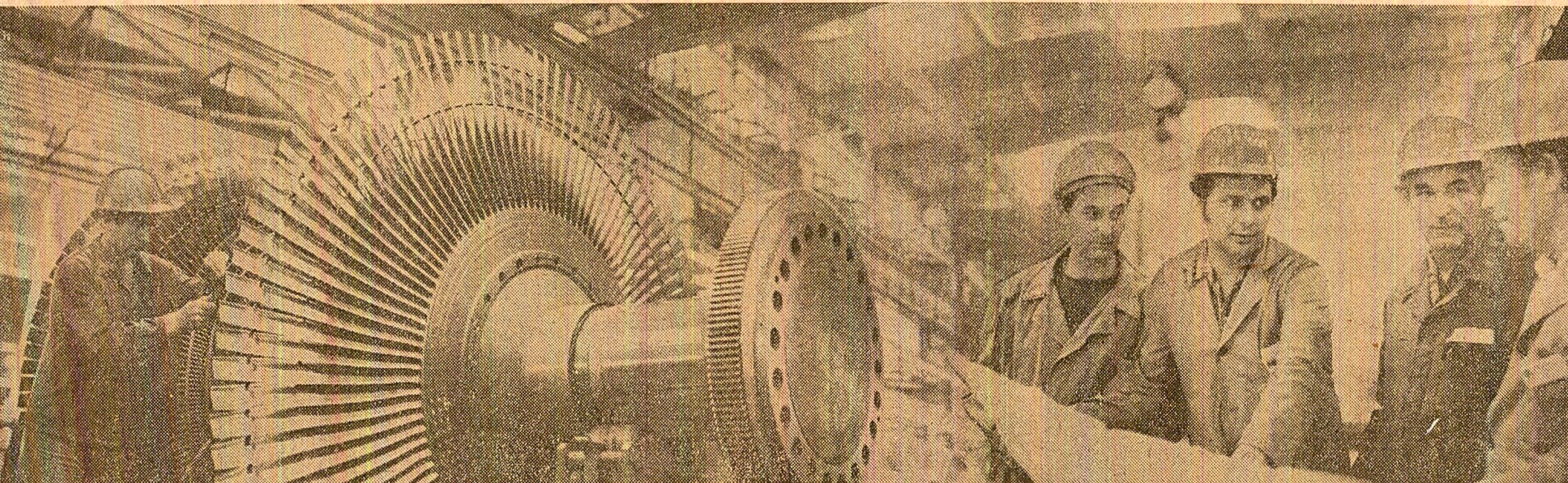
Numeroase din turbinele „cetăților luminii” ale țării s-au născut în această uzină. Ca și cea din prezenta fotografie, cu o putere de 330 MW. Iată și numele citorva din autorii turbinelor românești (de la stînga la dreapta): Zamfir Spulber, muncitor, Marin Tudor, șef de echipă, Alexandru Ghinescu, inginer, Simion Pipera, trasctor, Ion Florea, maistr
