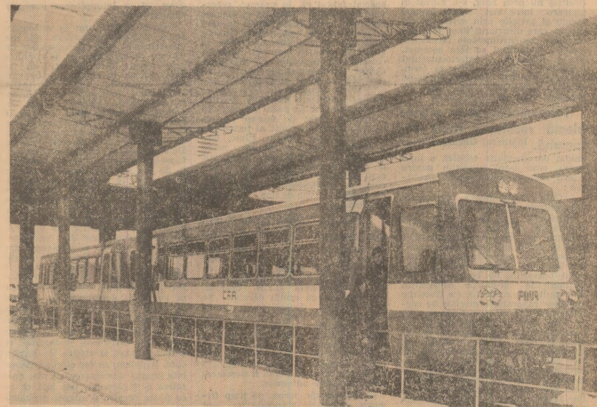
În aceste zile, la întreprinderea „23 August” din Capitală a ieșit de pe banda de montaj un nou tip de automobil de 200 CP (în fotografie), cu caracteristici tehnice superioare, destinat transportului de călători pe linii secundare și în zonele suburbane. Foto: R. Cristescu
