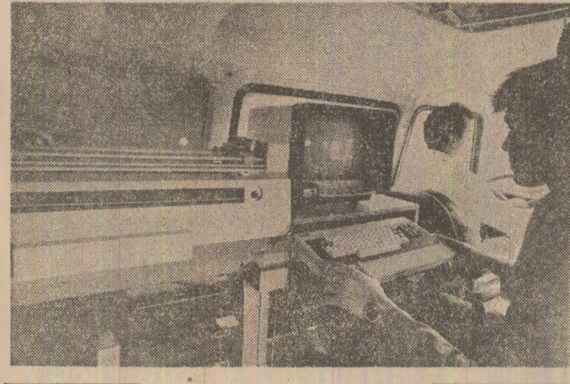
„Energobuzul” — un modern și eficient echipament mobil pentru diagnosticare exactă și operativă a consumurilor energetice. Dotat cu un complex echipament de calcul și cu o gamă variată de aparate de măsură și control, cu ajutorul „Energobuzului” se poate realiza o analiză energetică minuțioasă, care pune în evidență „robinetele” risipei de energie și combustibil din întreprinderi sau mari platforme industriale.
