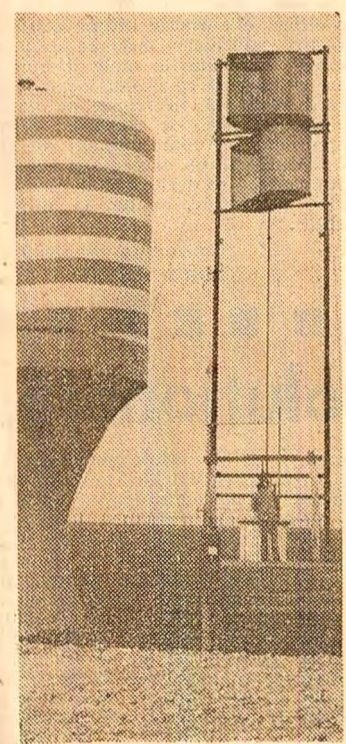
La ferma Vișina a I.A.S. Corabia funcționează o instalație eoliană pentru pomparea apei
