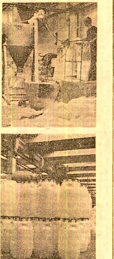
Muncitorii și specialiștii de la întreprinderea de prelucrare a maselor plastice din Năsăud au acumulat o valoroasă experiență în privința valorificării materialelor refozabile. În fotografia de sus: instalația realizată prin autodepozare pentru măcinarea foliei de polietilenă. În fotografia de jos: produse noi realizate în proporție de peste 90 la sută din mase plastice uzate. Foto: S. Cristian
