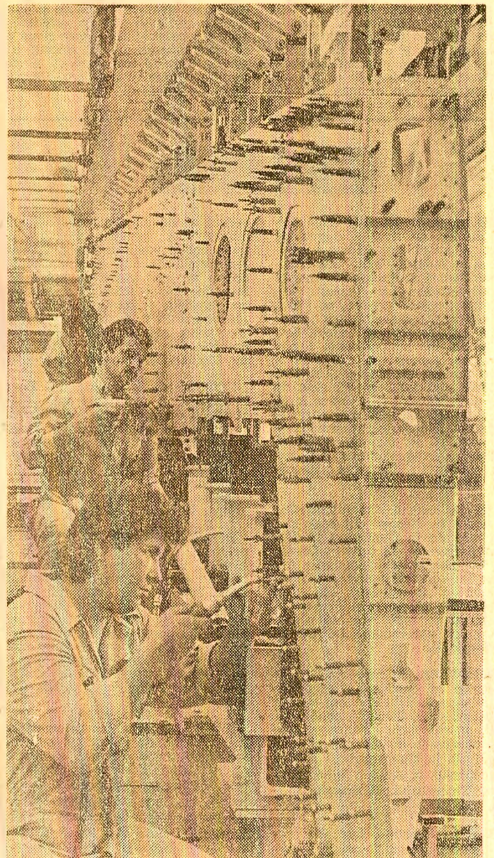
Muncă migăloasă, de înaltă calitate la construcția aripilor de avion
