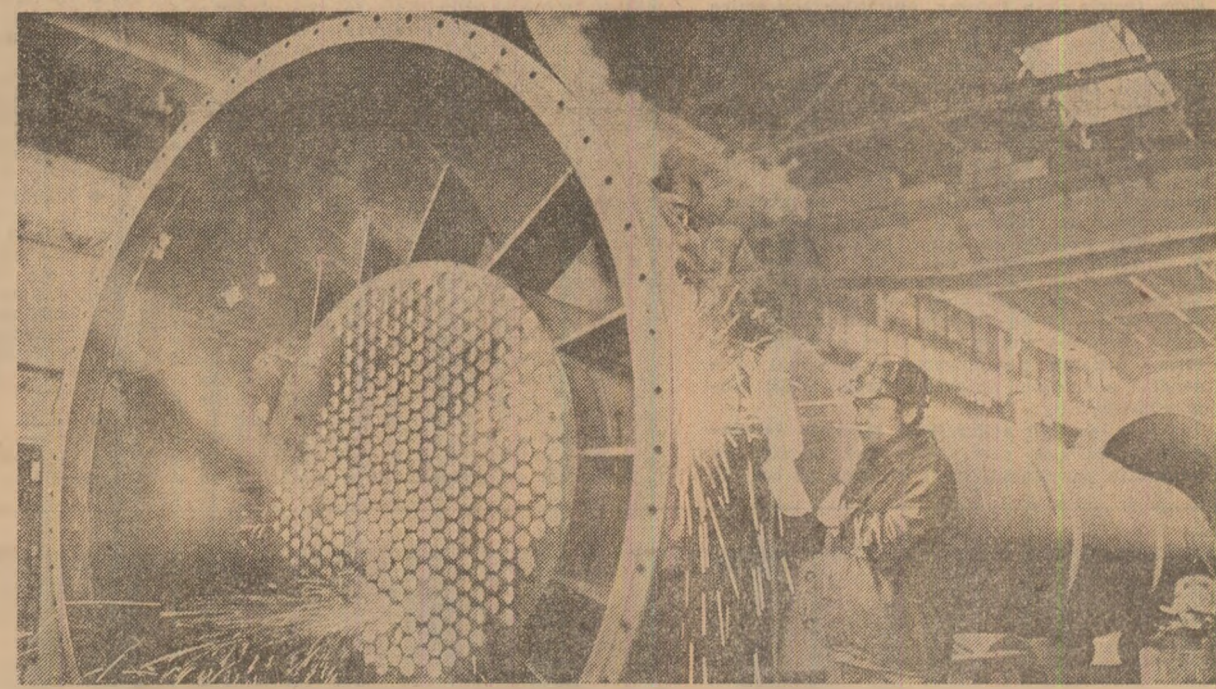
Întreprinderea de utilaj tehnologic din Buzău. Aspect din secția cazangerie grea. Foto: E. Dichseanu
