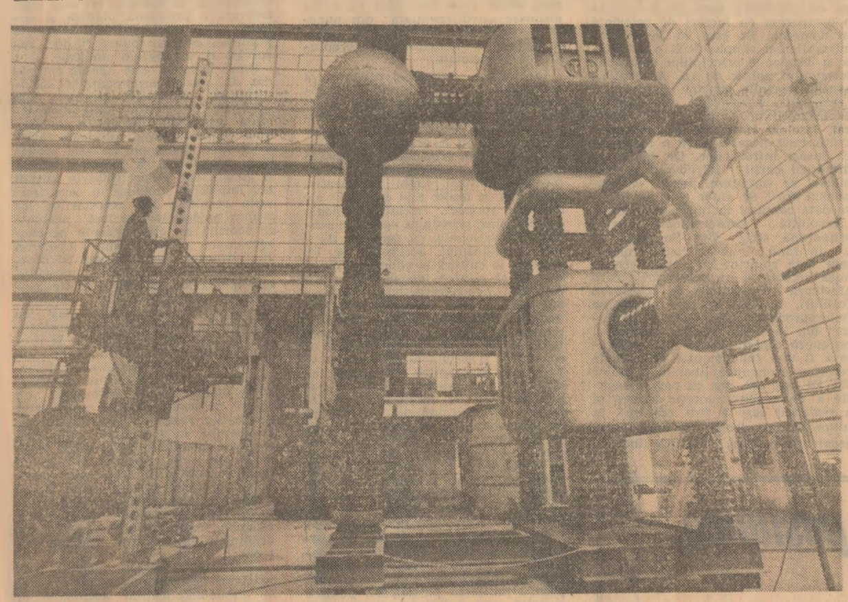
Aspect de la Uzina de reparat transformatori și aparat electric Roman. Foto: AGERPRES — M. Alexe
