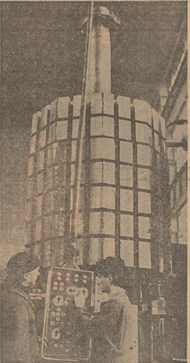
Intreprinderea constructoare de mașini Reșița. Aspect din secția mecanică grea, unde se prelucurează un nou rotor pentru turbine, ce va fi livrat în curînd beneficiarului. Foto: S. Cristian
