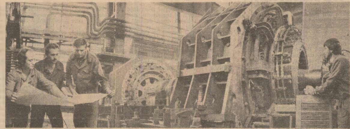
La întreprinderea constructoare de mașini din Reșița se lucrează la cel mai mare motor de curent continuu construit până acum în țară (de 5400 kW), destinat industriei metalurgice. Foto: Eugen Dichiseanu
