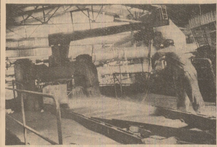
Întreprinderea „Laminorul” din Brăila; aspect de la laminorul nr. 2. Foto: E. Dichiseanu
