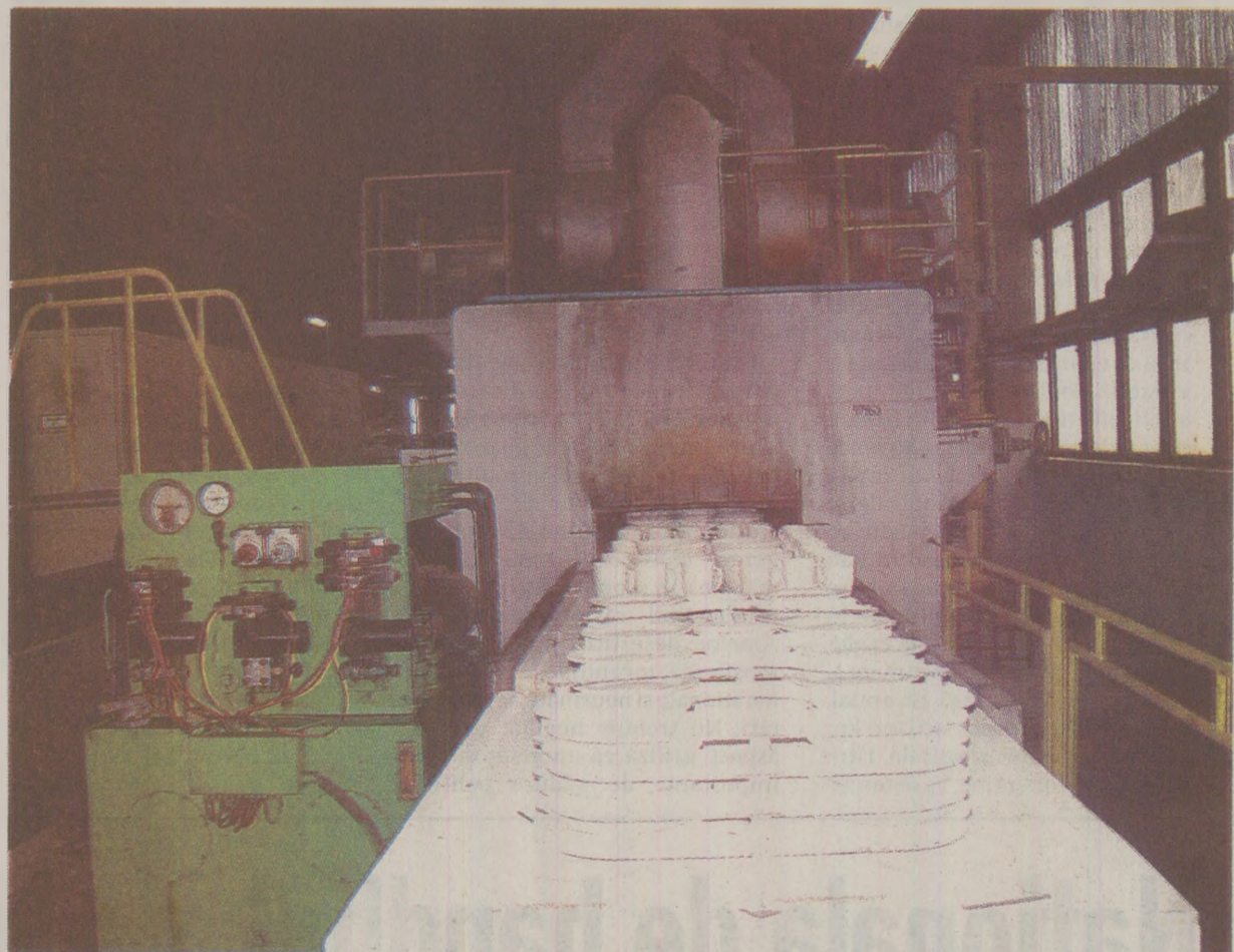
Cuptorul cu ardere rapidă a masei de porțelan a fost construit ca urmare a unei necesități de modernizare tehnologică
