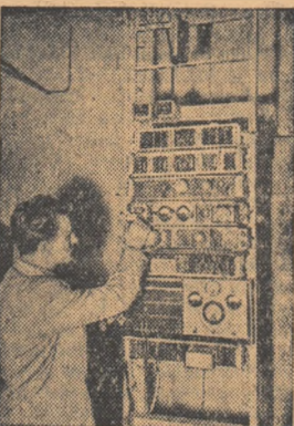
Tovarășul Barbu Enea, lector la Institutul politehnic din București, verifică noua stație de releu, creată la acest Institut, înainte de a o pune în funcțiune.
