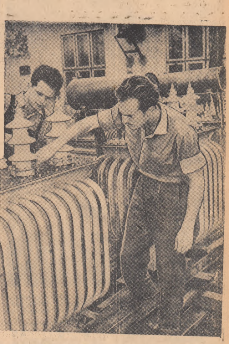
Produsele finite de uz medicinal cit și industrial, fabricate la întreprinderea „Electrotehnică” din Capitală au ajuns să fie cunoscute și apreciate calitativ atât în țară cit și peste hotare. În fotografie: doi dintre tehnicienii de înaltă calificare ai fabricii efectuînd o ultimă verificare la un lot de transformatori.
