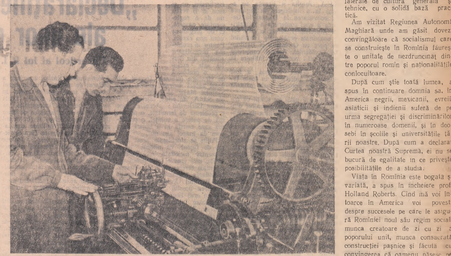
Maestrul Dumitru Tiron și regorul Ștefan Abodi din secția carde a întreprinderii „Encsel Mauriciu” din Tg. Mureș sînt frunțași în muncă. Iată-i în fotografie controlînd elasticitatea șocabei mașinii de confecționare capace carde de bumbac.
