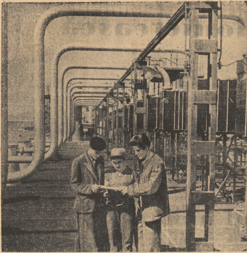
Ing. B. Weisbuch împreună cu operatorul Vasile Someșanu și lucrătorul Rada Neacșu examinând parametrii procesului la instalația de acid clorhidric de la Combinatul chimic Borzești. Foto: A. VIERU
